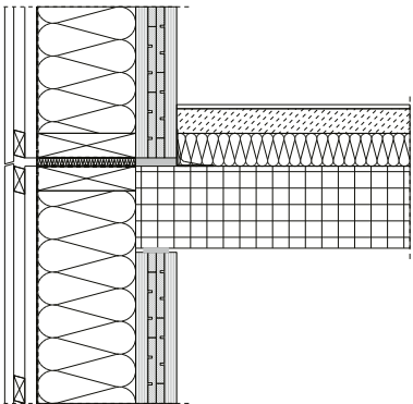
Anschlussdetail (vert.) – Geschossübergang
