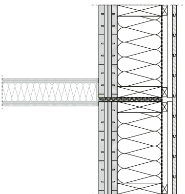
Anschlussdetail (horz.) – Elementfuge an Trockenbau
