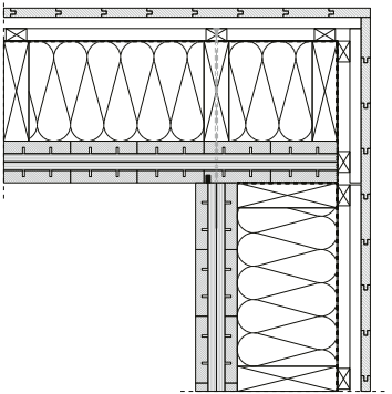
Eckdetail (horz.) – Elementfuge
