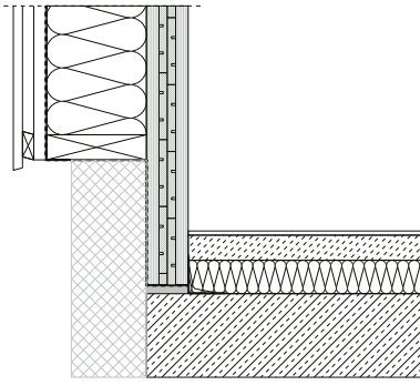
Anschlussdetail (vert.) – Sockelbereich
