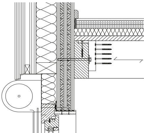
Beispiel: Detailanschluss Holzbalkendecke an Außenwand mit NHT-Verbinder
