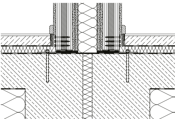
Beispiel: Gebäudetrennwand
