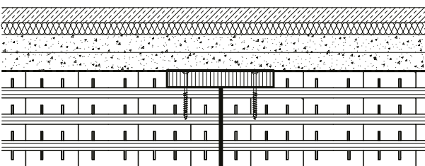
Beispiel: Deckenstoß, Deckleiste oben
