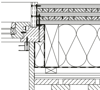
Beispiel: Fensteranschluss Horizontalschnitt sowie Einbau Leerdose
