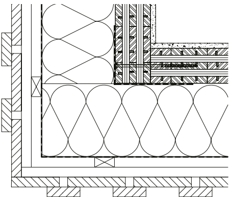
Beispiel: Eckverbindung Außenwand
