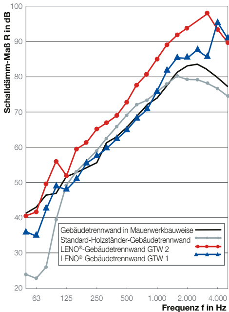
Quelle: Holtz, F., Hessinger, J., Rabold A., u. a.: INFORMATIONSDIENST HOLZ, holzbau handbuch, R3/T3/F4, Schallschutz Wände und Dächer, Hrsg. Holzabsatzfonds u. DGfH, Bonn/München 2004
