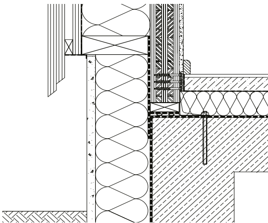
Beispiel: Sockeldetail, Perimeterdämmung nach oben gezogen
