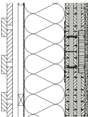
Beispiel: Wandstoß mit oberflächenbündiger Stoßdeckungsleiste
