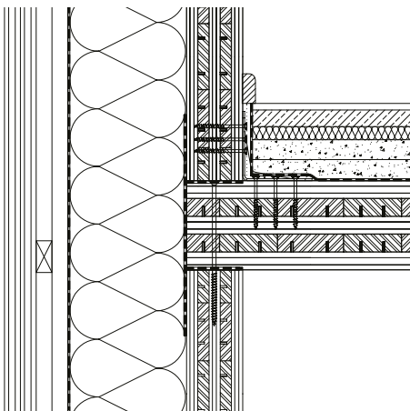
Beispiel: Detailanschluss LENO®-Decke an geschosshoher Außenwand
