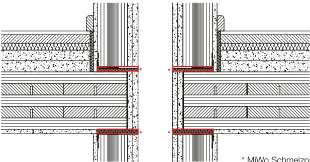
Beispiel: Deckenanschluss Gebäudetrennwand
