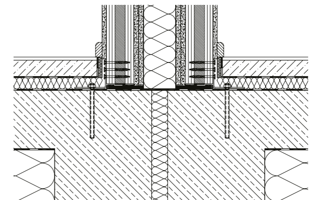
Beispiel: Gebäudetrennwand
