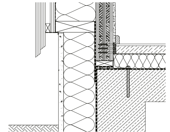
Beispiel: Sockeldetail, Perimeterdämmung nach oben gezogen
