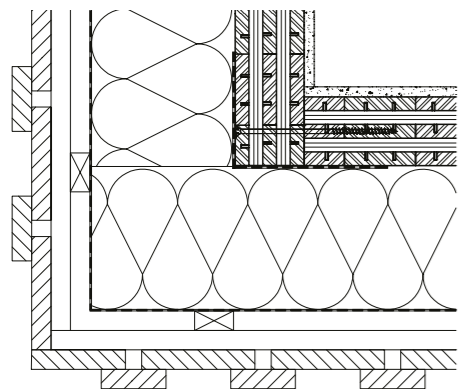
Beispiel: Eckverbindung Außenwand
