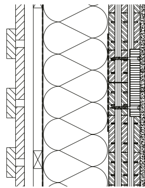
Beispiel: Wandstoß mit oberflächenbündiger Stoßdeckungsleiste
