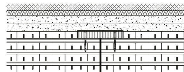
Beispiel: Deckenstoß, Deckleiste oben
