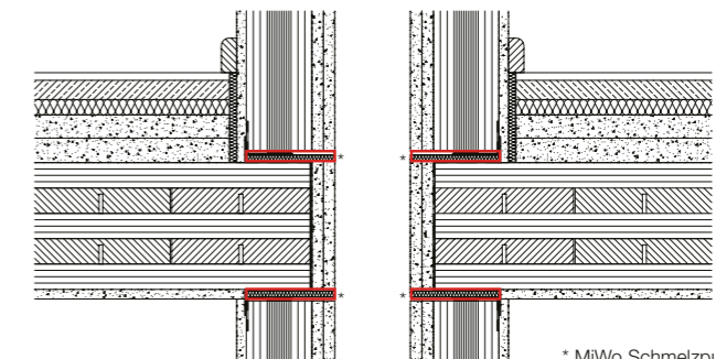
Beispiel: Deckenanschluss Gebäudetrennwand
