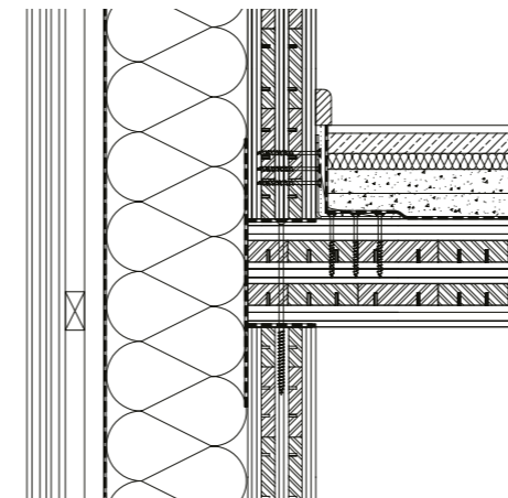
Beispiel: Deckenstoß, Deckleiste oben
