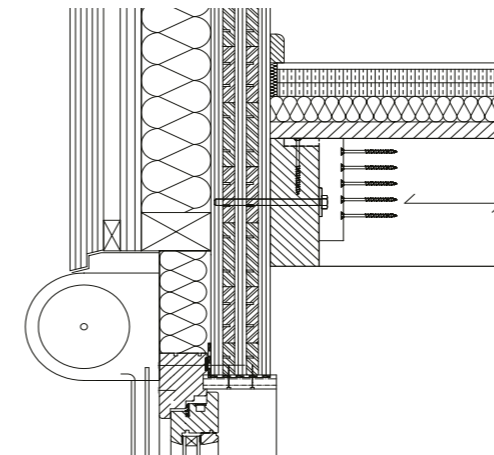
Beispiel: Detailanschluss LENO®-Decke an geschosshoher Außenwand
