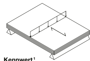
Spannrichtung parallel zur Faserrichtung der Decklagen
