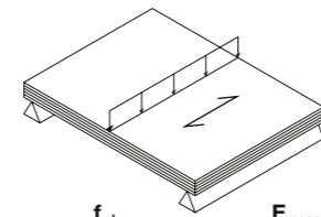
Spannrichtung senkrecht zur Faserrichtung der Decklagen
